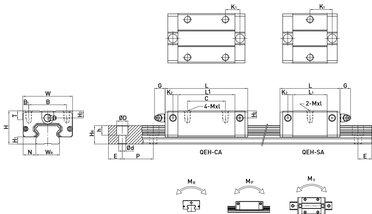
2-7-9 QE系列直线导轨尺寸表 (1) QEH-CA / QEH-SA
