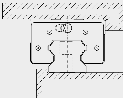
单支滑轨有承靠面配置
