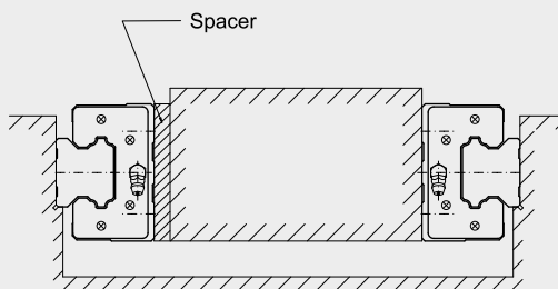
背向两支滑轨配置
