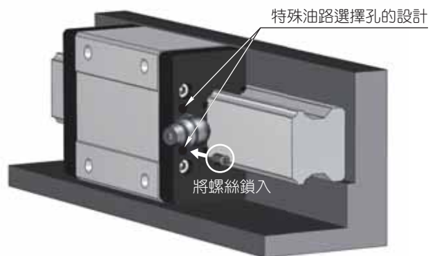
圖2.2.8 油路選擇孔
