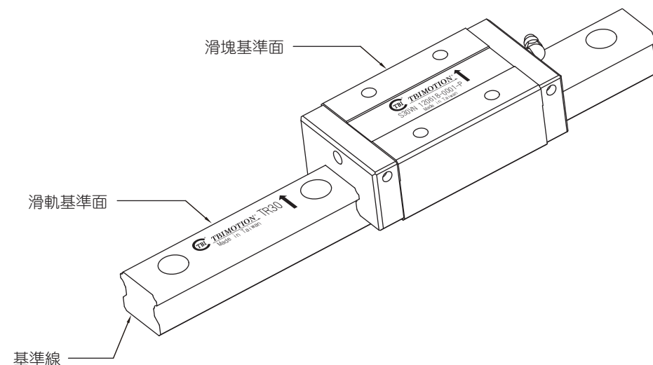
圖1.11.1 基準面的表示
