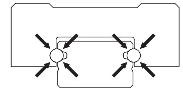
圖2.3.4 哥德式45°四方向負荷結構
