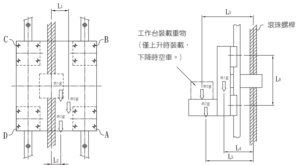
圖1.8.4 使用條件
