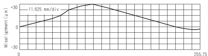
圖1.9.3 直線度誤差的形狀
