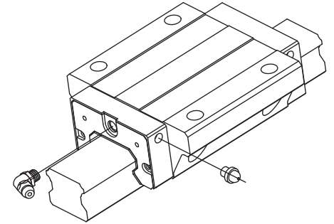
圖2.2.7 油嘴位置
