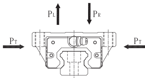
圖1.6.3 滑軌的負荷方向、力矩方向
