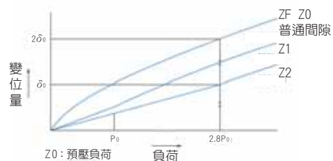
圖1.10.2 剛性數據
