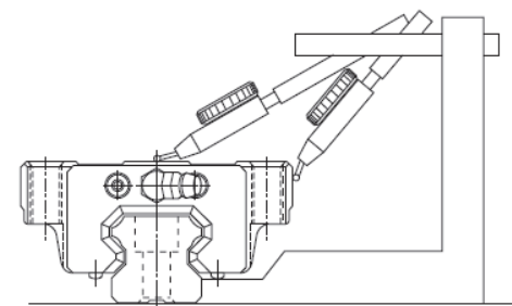
圖1.9.1 行走平行度
