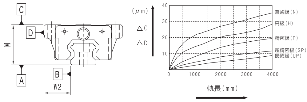
圖2.2.5 精度標準
