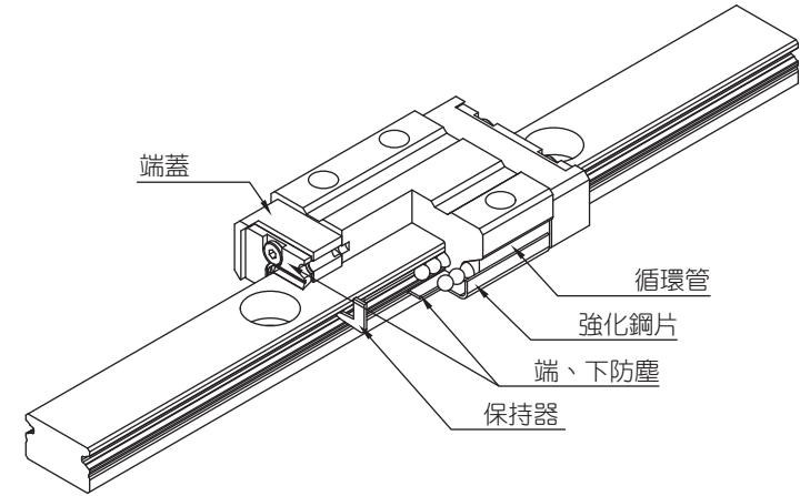
圖2.3.5 TM本體結構
