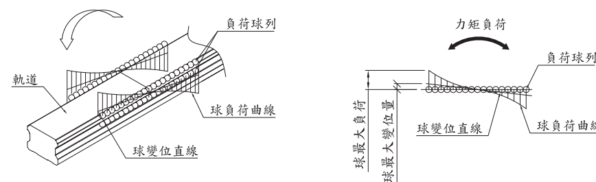
圖1.6.1 力矩作用時球的負荷
