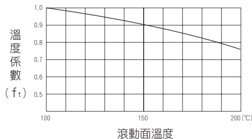
圖1.3.3 溫度係數 (f t )
