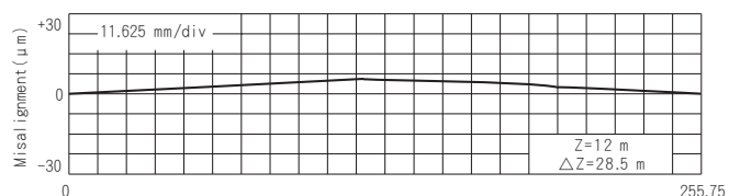
圖1.9.4 工作台的水平變位
