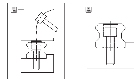
圖2.2.15 滑軌防塵方式
