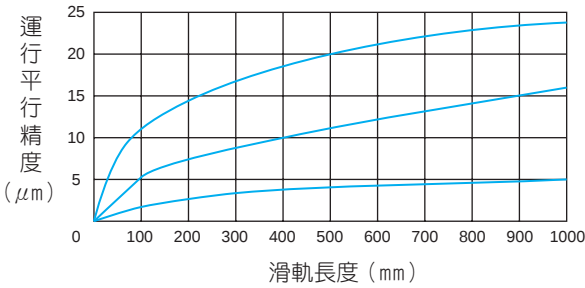
圖2.3.6 滑塊相對於滑軌基準面之運行平行精度
