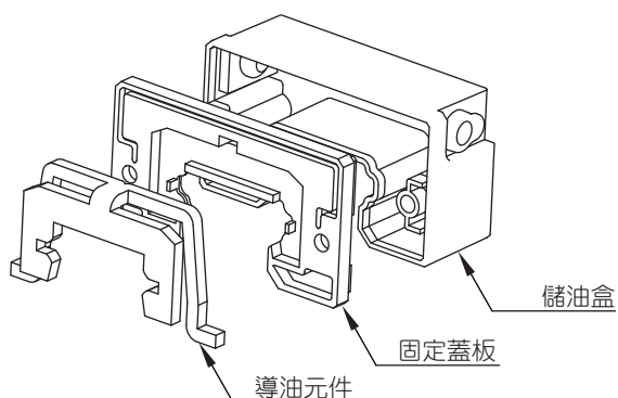
圖2.2.14 自潤式油箱構造
