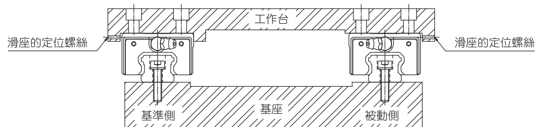
圖 1.11.12 基準側滑軌沒有定位螺絲的情況
