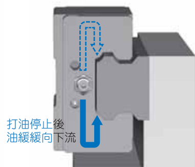
圖2.2.10 停止打油後油品流向
