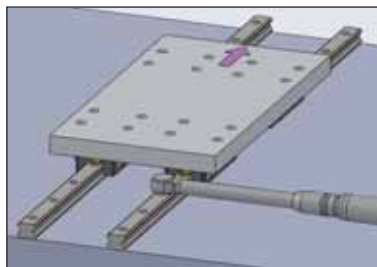
圖1.11.16 仿效基準側軌道的方法
