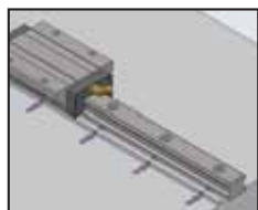
圖 1.11.9 安裝的檢查
