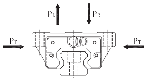
圖1.6.5 滑軌的等效負荷
