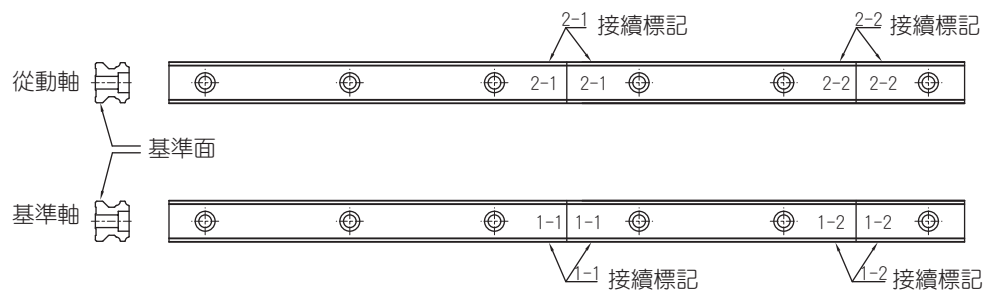
圖1.11.3 滑軌接牙標示
