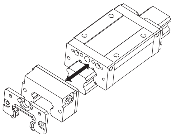
圖2.2.13 自潤式油箱組件方式
