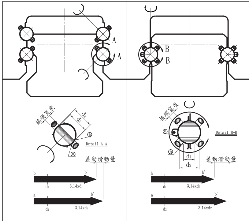
圖1.1.1 四排鋼珠等負荷設計
