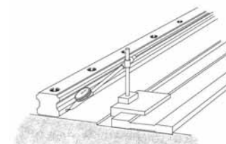
圖1.11.20 用直線塊規的方法
