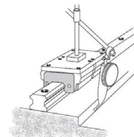
圖1.11.19 利用假基準面的方法
