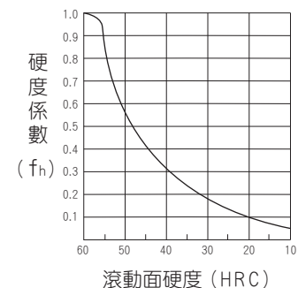
圖1.3.2 硬度係數 (f h )
