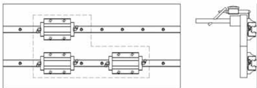
圖1.11.15 移動工作台的方法
